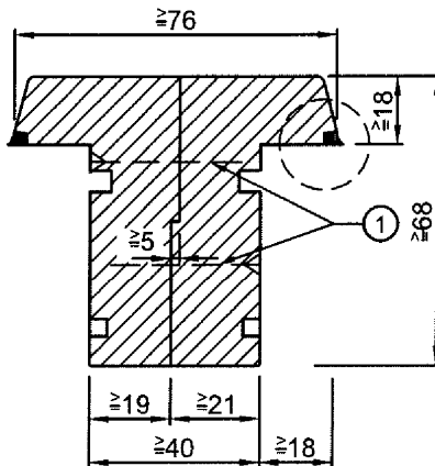
Falz-Verbindung
