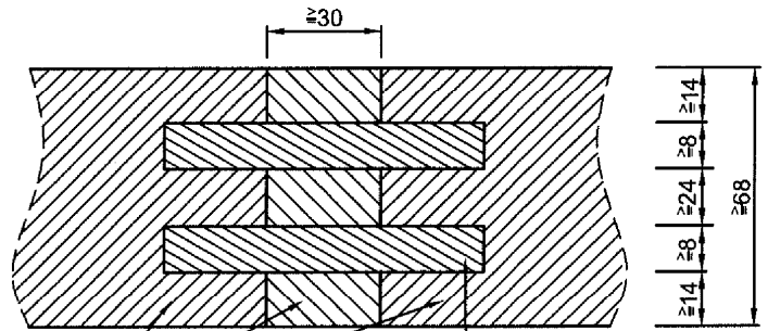
Holzdübel aus LH
