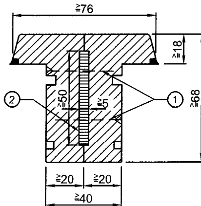
Flachfeder-Verbindung
