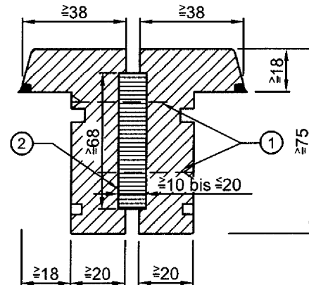
Schattennut-Verbindung
