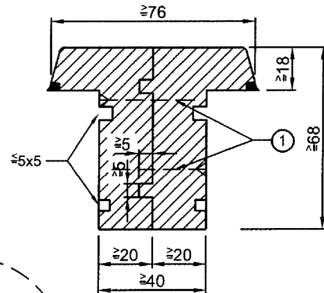
Zapfen-Verbindung
